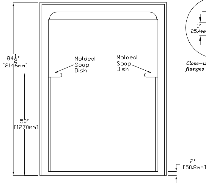
ELEVATION
